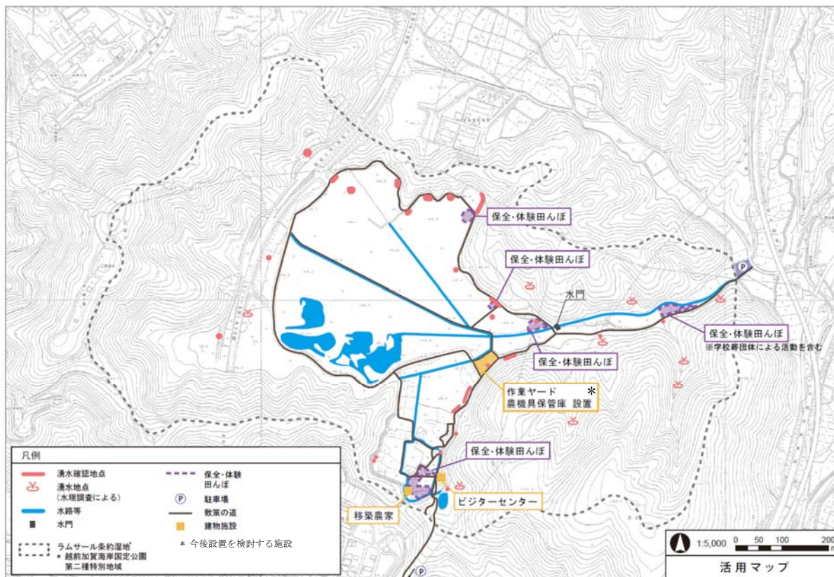
図 施設配置計画図（既存の施設も含む）
